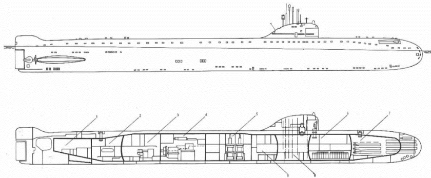
Опытная подводная лодка проекта 627 (1958 год): а — боковой вид; б — продольный разрез.
