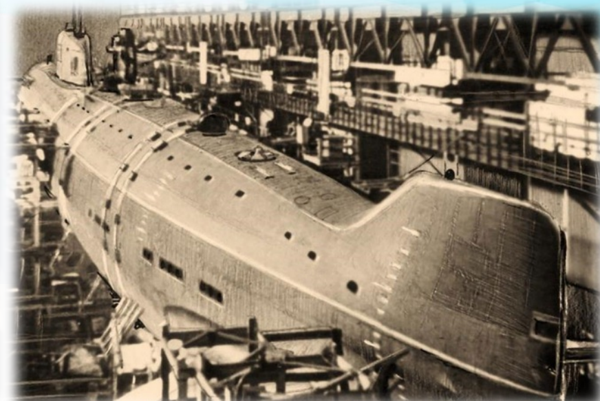
НА СТАПЕЛЕ ЦЕХА №42 СУДОСТРОИТЕЛЬНОГО ЗАВОДА № 402. КОРМОВАЯ ЧАСТЬ
