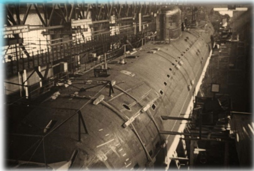
НА СТАПЕЛЕ ЦЕХА №42 СУДОСТРОИТЕЛЬНОГО ЗАВОДА № 402. НОСОВАЯ ЧАСТЬ
